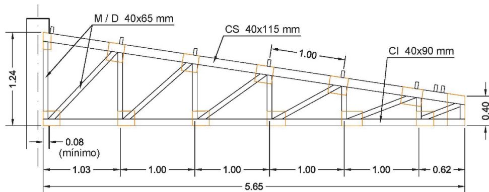
ESTRUCTURA RETICULADA 1
