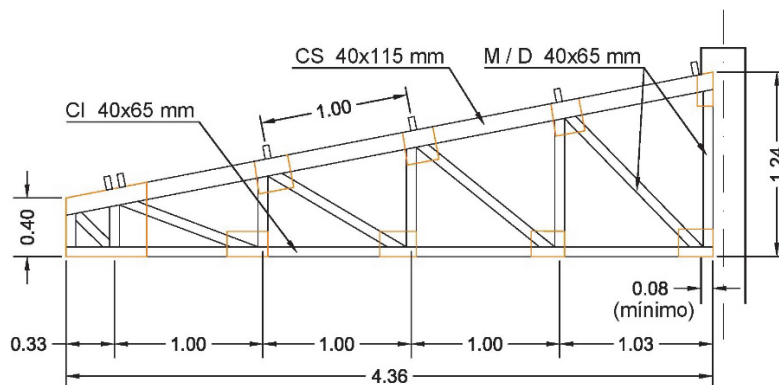
ESTRUCTURA RETICULADA 2
