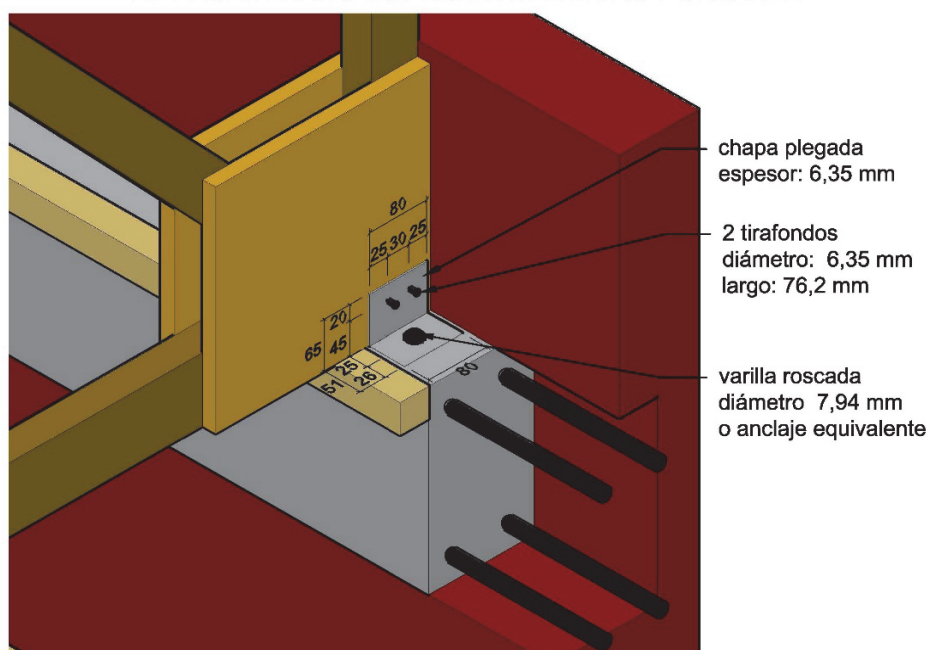
DETALLE DE UNIÓN DE LA CABIADA AL ENCADENADO SUPERIOR DEL MURO PORTANTE
